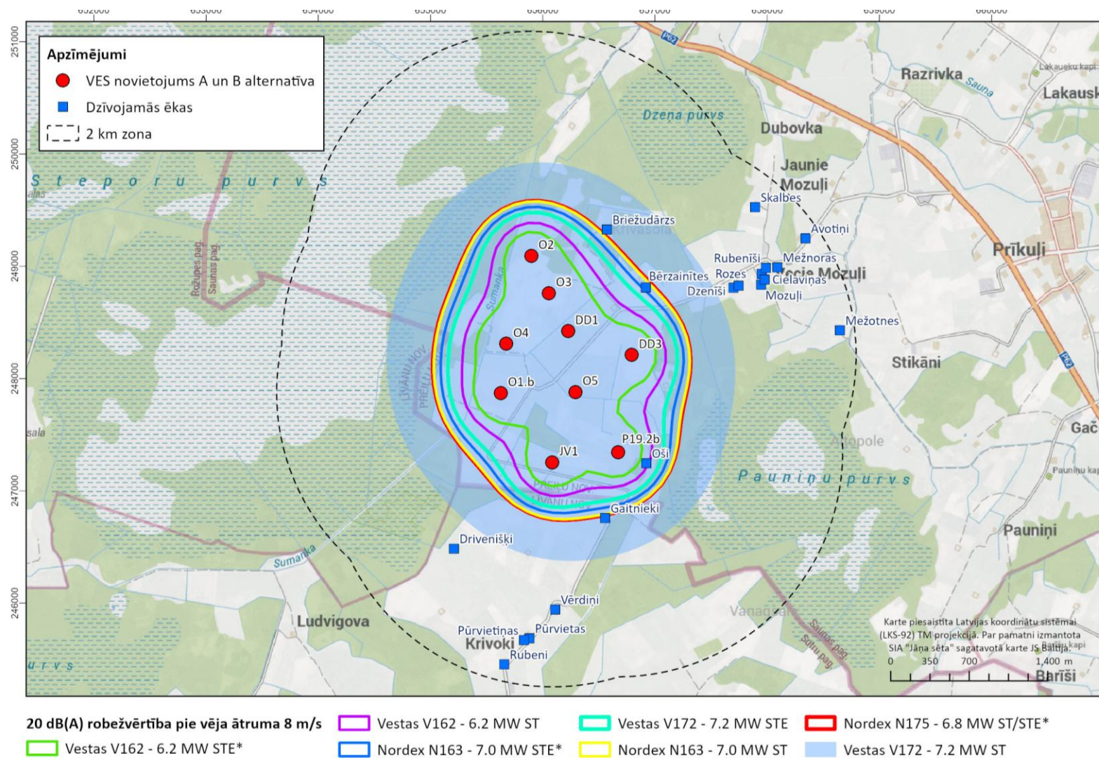
3.1.18. attēls. Zemas frekvences trokšņa virs 20 dB(A) ietekmes zona pie vēja ātruma 8 m/s – A un B alternatīva dienvidu daļa
