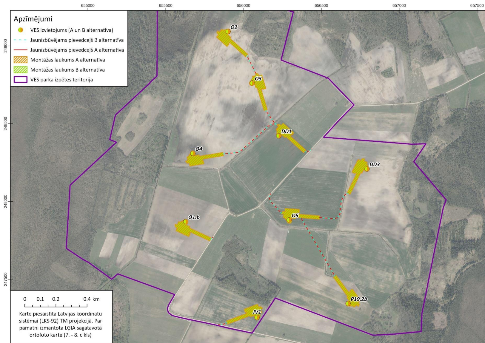
2.5. attēls. Jaunbūvējamo pievedceļu un laukumu novietojums vēja parka "Pīrkulī" dienvidu daļā
