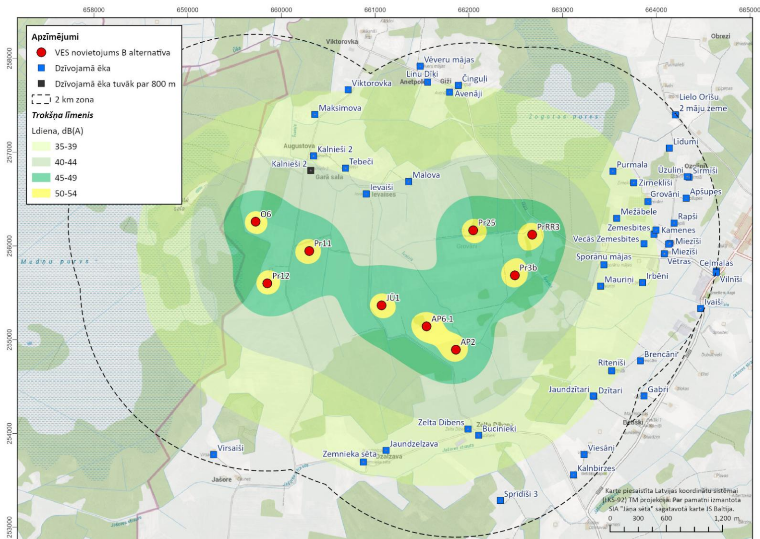
3.1.8. attēls. Vestas V172 – 7.2 MW ar standarta spārnem radītais trokšņa līmenis paredzētās darbības apkārtnē vides trokšņa rādītājam L_{diena} – B alternatīva ziemeļu daļa
