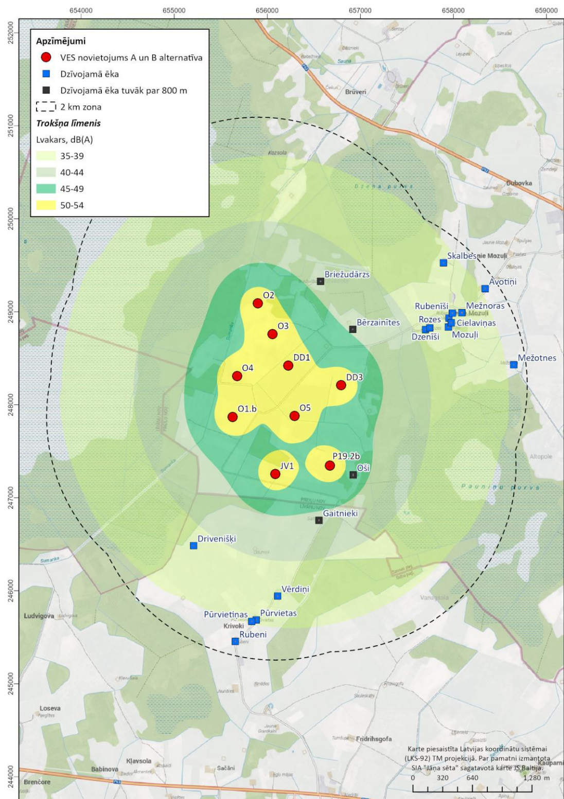
3.1.13. attēls. Vestas V172 – 7.2 MW ar standarta spārniem radītais troksņa līmenis paredzētās darbības apkārtnē vides troksņa rādītājam L_{vakars} A un B alternatīva dienvidu daļa
