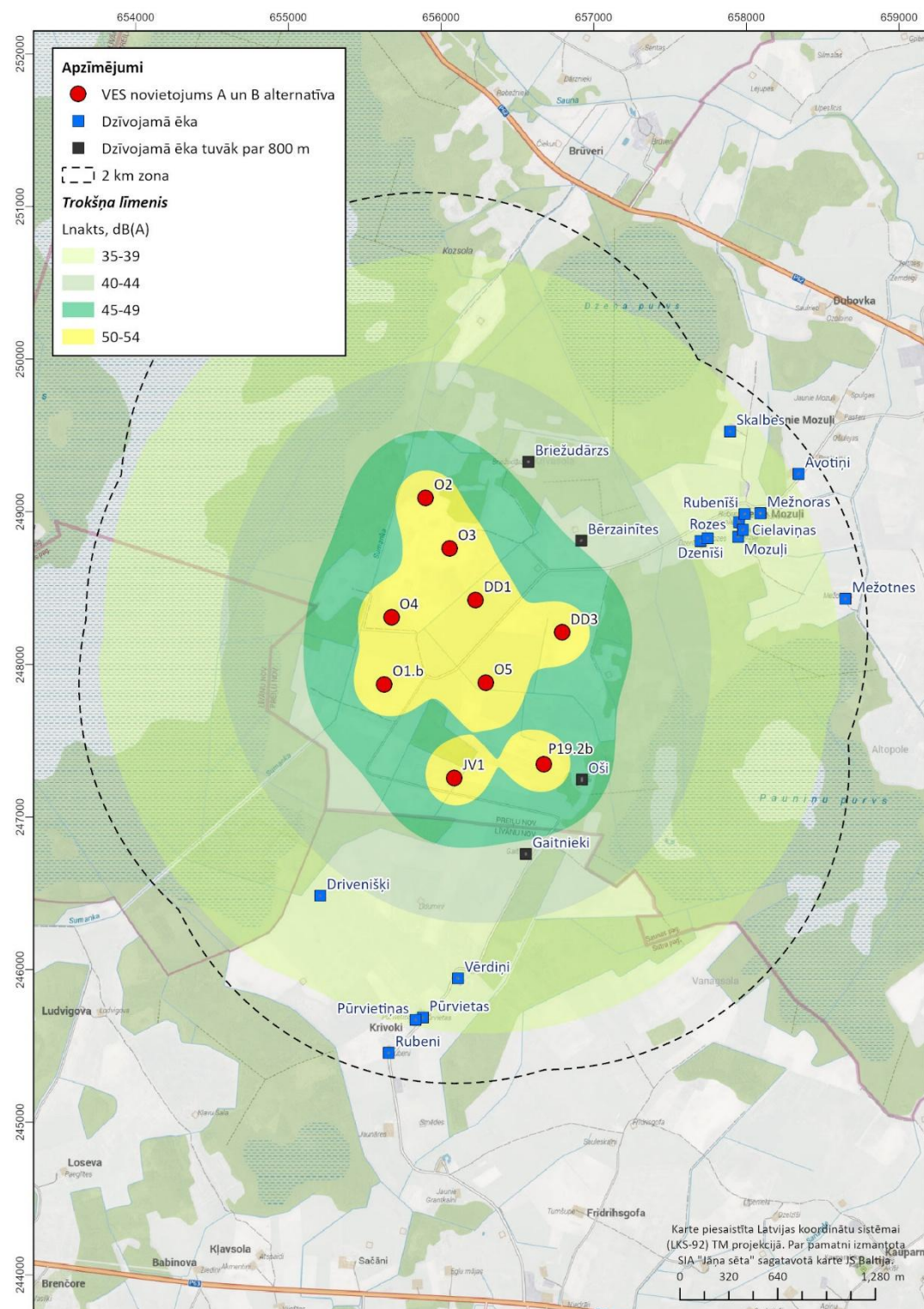
3.1.14. attēls. Vestas V172 – 7.2 MW ar standarta spārniem radītais trokšņa līmenis paredzētās darbības apkārtņē vides trokšņa rādītājam L_{nakts} A un B alternatīva dienvidu daļa
