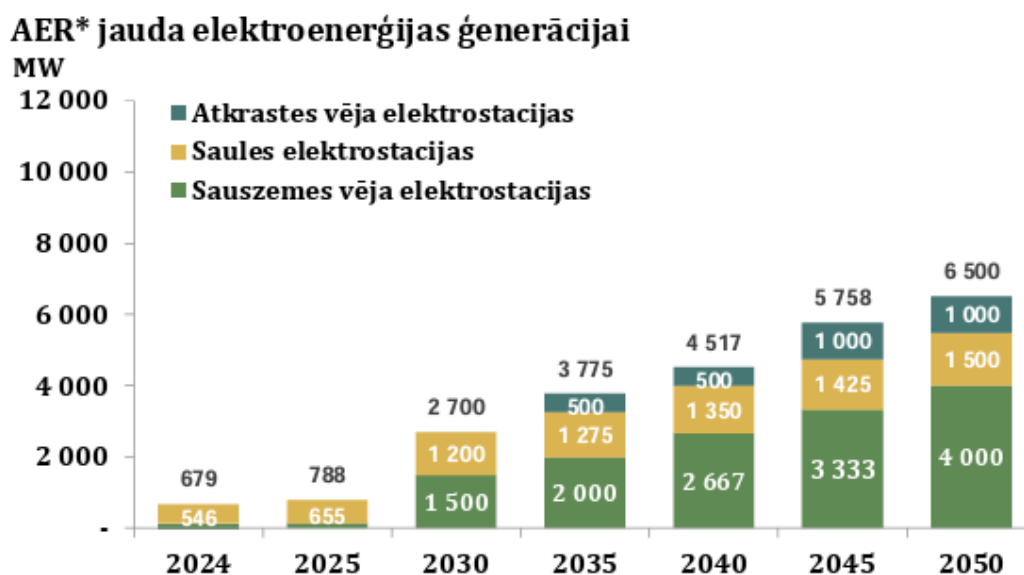
3.12.10. attēls. AER uzstādītās jauda elektroenerģijas ģenerācijai prognoze Bāzes scenārijā, *izņemot HES 347
