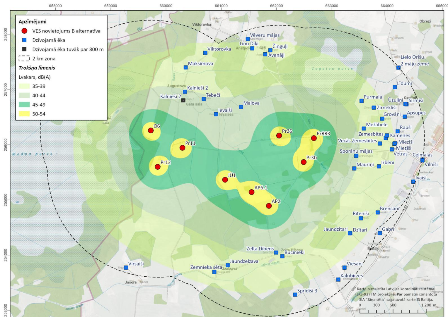
3.1.9. attēls. Vestas V172 – 7.2 MW ar standarta spārniem radītais troksņa līmenis paredzētās darbības apkārtnē vides troksņa rādītājam Lvakars – B alternatīva ziemeļu daļa
