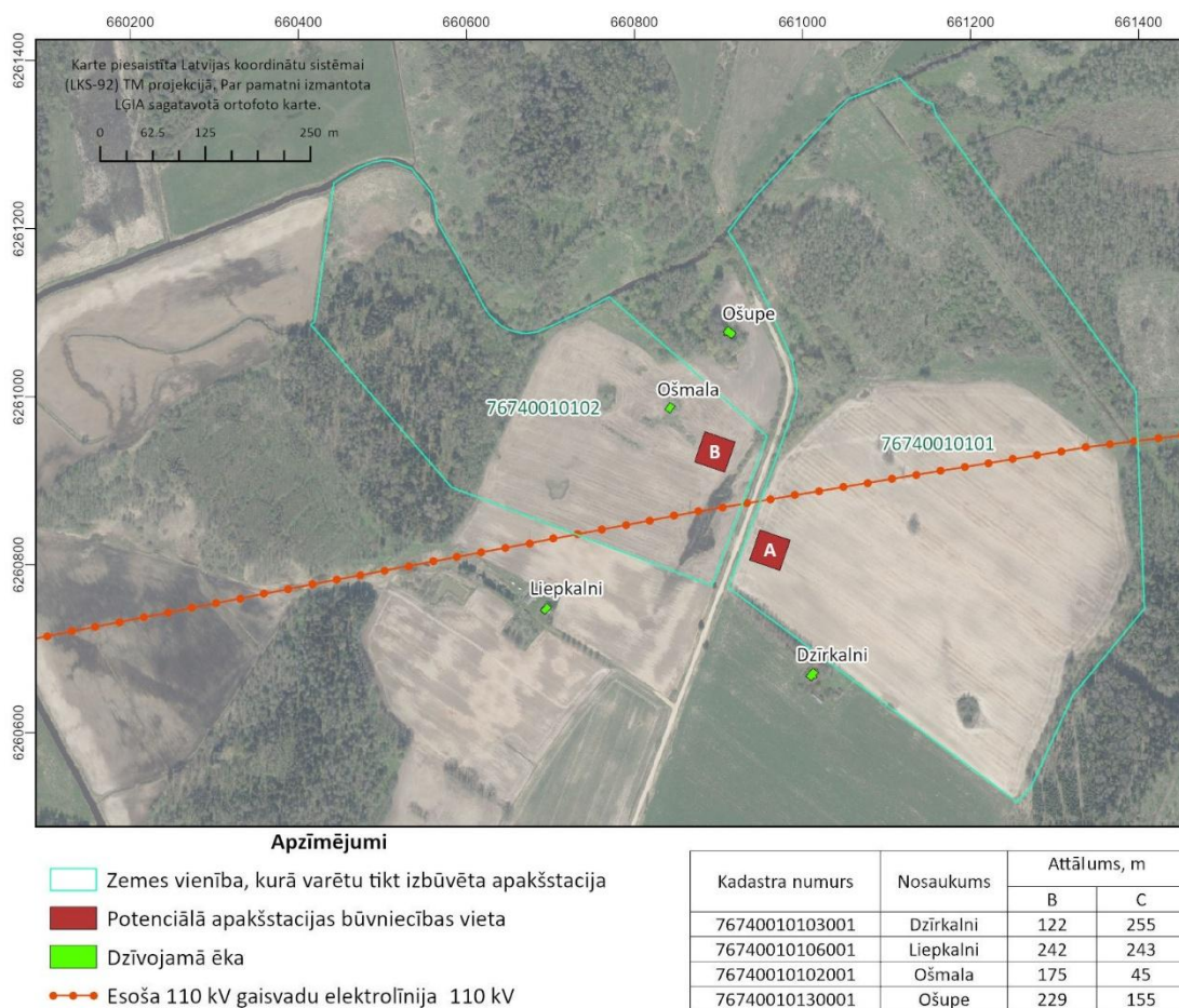
3.1.3. attēls. Potenciālā apakšstacijas būvniecības vieta – A un B alternatīva
