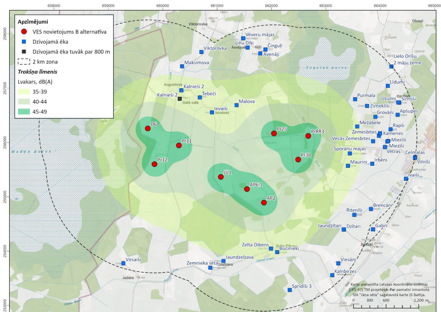
3.1.24. attēls. Nordex N175 – 6.8 MW ar aerodinamiski uzlabotiem spārnēm radītais trokšņa līmenis paredzētās darbības apkārtnē vides trokšņa rādītājam L_{vakars} – B alternatīva ziemeļu daļa
