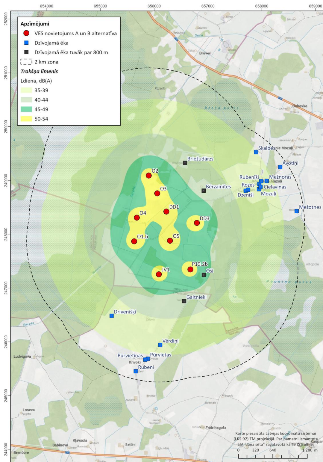
3.1.12. attēls. Vestas V172 – 7.2 MW ar standarta spārniem radītais trokšņa līmenis paredzētās darbības apkārtnē vides trokšņa rādītājam L_{diena} A un B alternatīva dienvidu daļa
