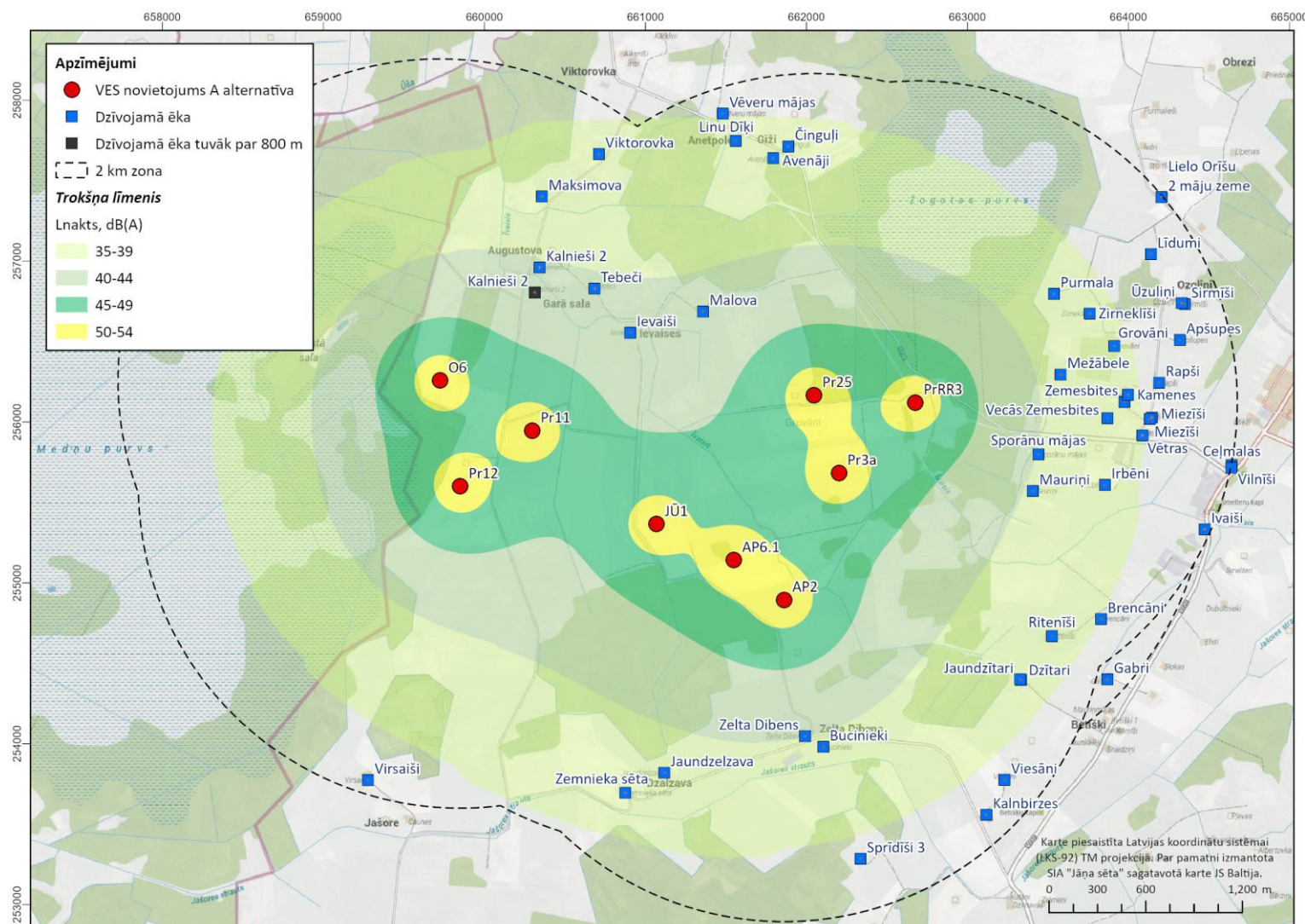
3.1.6. attēls. Vestas V172 – 7.2 MW ar standarta spārniem radītais trokšņa līmenis paredzētās darbības apkārtnē vides trokšņa rādītājam L_{nakts} – A alternatīva ziemeļu daļa
